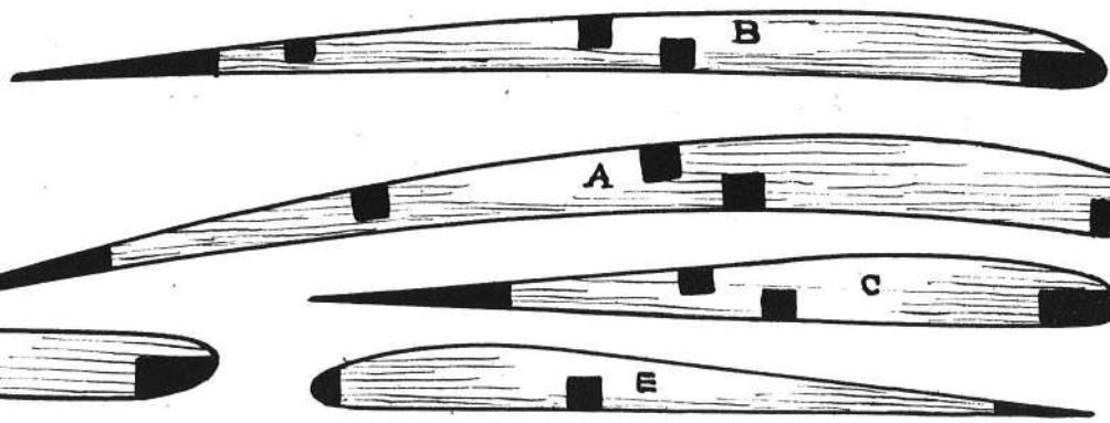
CENTINE DELL'ALA E DEL PIANO ORIZZONTALE IN SCALA 1:1
