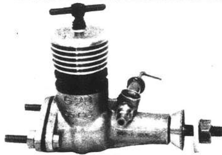
G. 28 - Cilindrata 0,5 cc. Corsa mm. 8,5. Alesaggio mm. 8,5. Peso gr. 38. Tipo diesel e tipo glow-plug. Regime di rotazione 15.000 giri con elica da 13x7,5.
