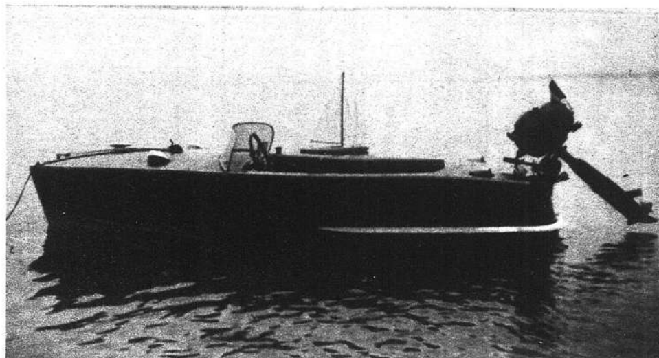
Questo è un motoscafo un po' più grosso: il « Libeccio », costruito da Vincenzo Ciri su disegno del torinese Corsi. Lunghezza m. 3,60; peso kg. 200; velocità, con motore da 25 HP, kmh. 52. Il cutter sullo sfondo denota la passione modellistica del costruttore
