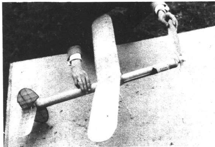
Un interessante modello Wakefield tedesco, costruito da Walter Spiegel, di Heidelberg. Caratteristica essenziale la fusoliera in tubo di balsa, alla quale l'ala viene fissata a mezzo di un appoggio costituito da due listelli
