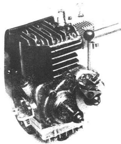
Un interessante motore a 4 tempi, a valvole laterali, costruito dal nostro collaboratore Giuseppe Tortora, e destinato ad un motoscafo radioguidato. Caratteristiche principali: alesaggio 25 mm., corsa 28 mm., cilindrata 13,7 cc. Lubrificazione a sbattimento; raffreddamento forzato a mezzo ventola; albero a gomiti e albero degli eccentrici montati su cuscinetti a sfere; velocità massima di rotazione 6.000 giri al minuto.
