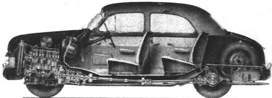
Nel titolo: La Fiat Nuova 1100-103. Sopra: vista in sezione della Fiat 1400
